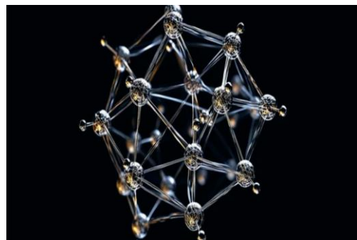
Salzatomstruktur
